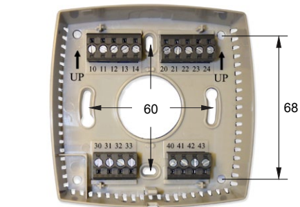
Figur 3. Bottenplatta med monteringsalternativ och plintarnas placering (mått i mm)
