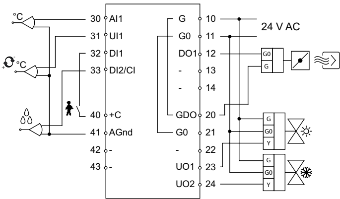
Figur 4. Inkopplingsschema för RC-H
