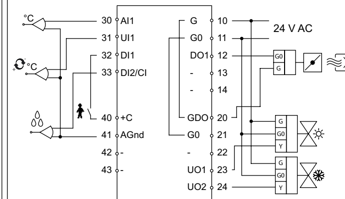
Figure 4. Schéma de connexion de RC-H
